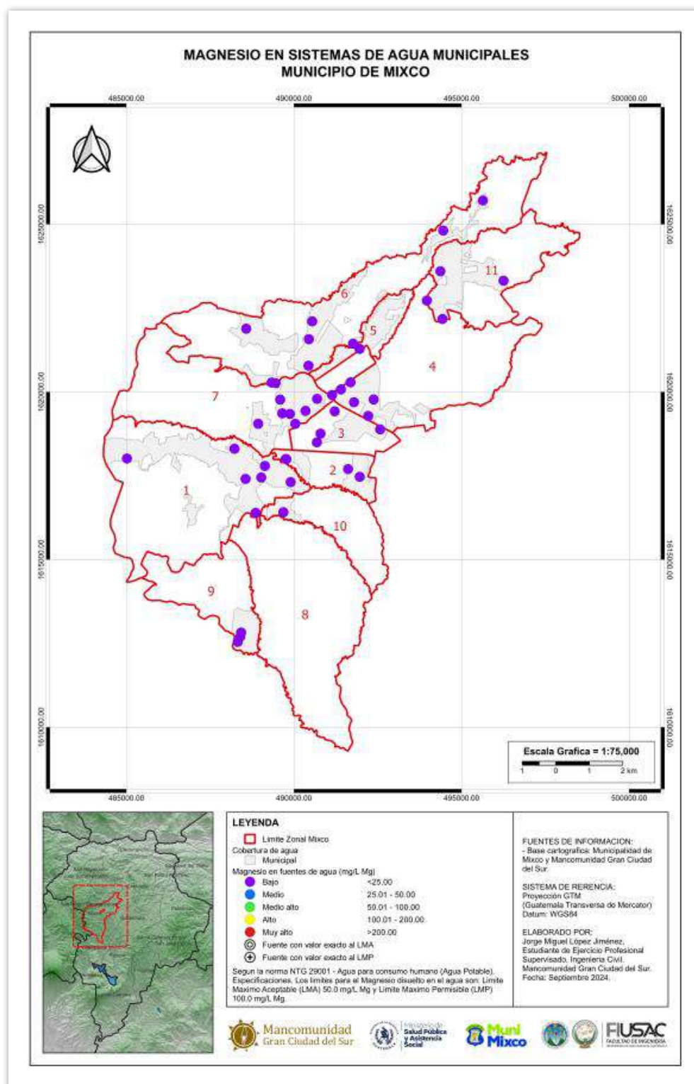
Mapa 39 – Magnesio disuelto en sistemas de agua municipales
