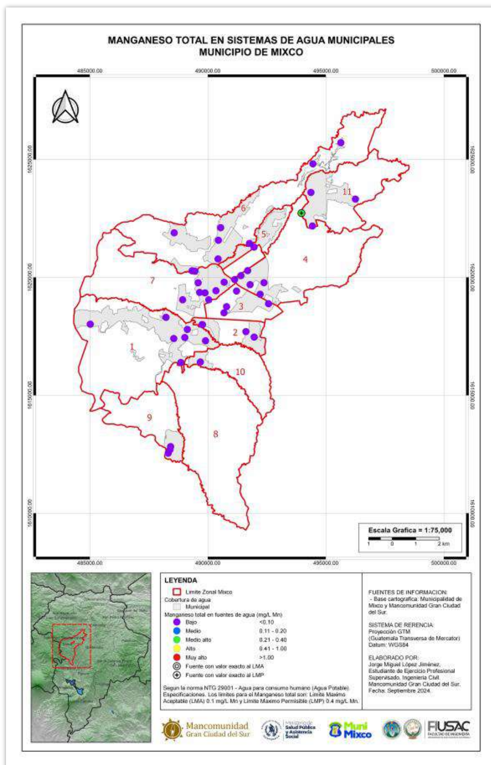
Mapa 31 – Manganeseo total disuelto en sistemas de agua municipales
