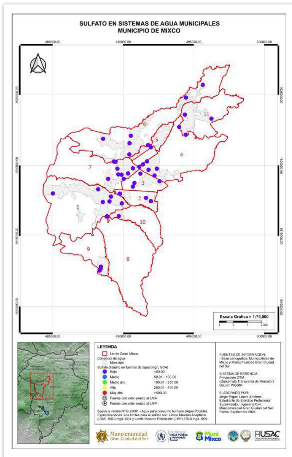
Mapa 34 – Sulfato disuelto en sistemas de agua municipales
