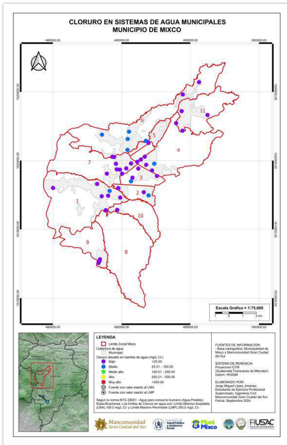
Mapa 36 – Cloruro disuelto en sistemas de agua municipales
