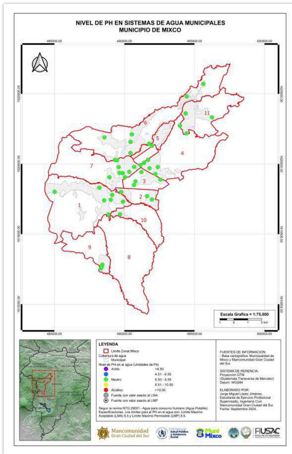
Mapa 41 – PH del agua en fuentes de agua municipales
