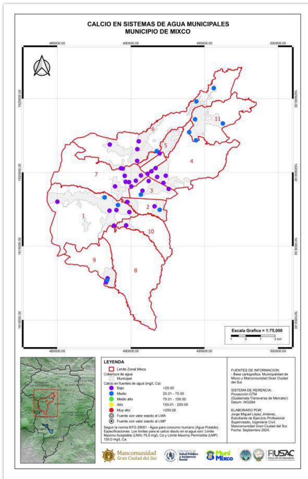
Mapa 38 – Calcio disuelto en sistemas de agua municipales
