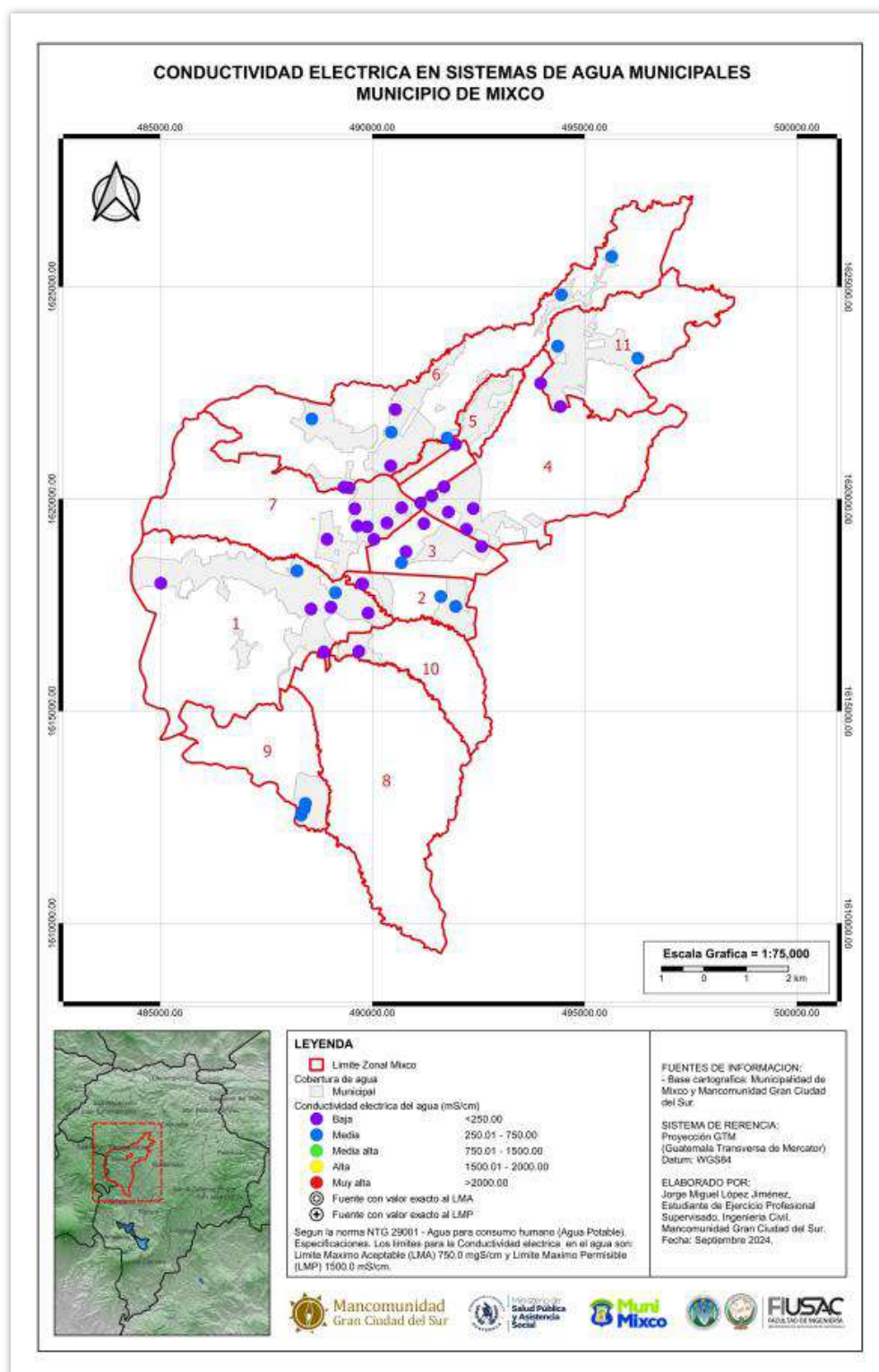
Mapa 40 – Conductividad eléctrica del agua en sistemas de agua municipales
