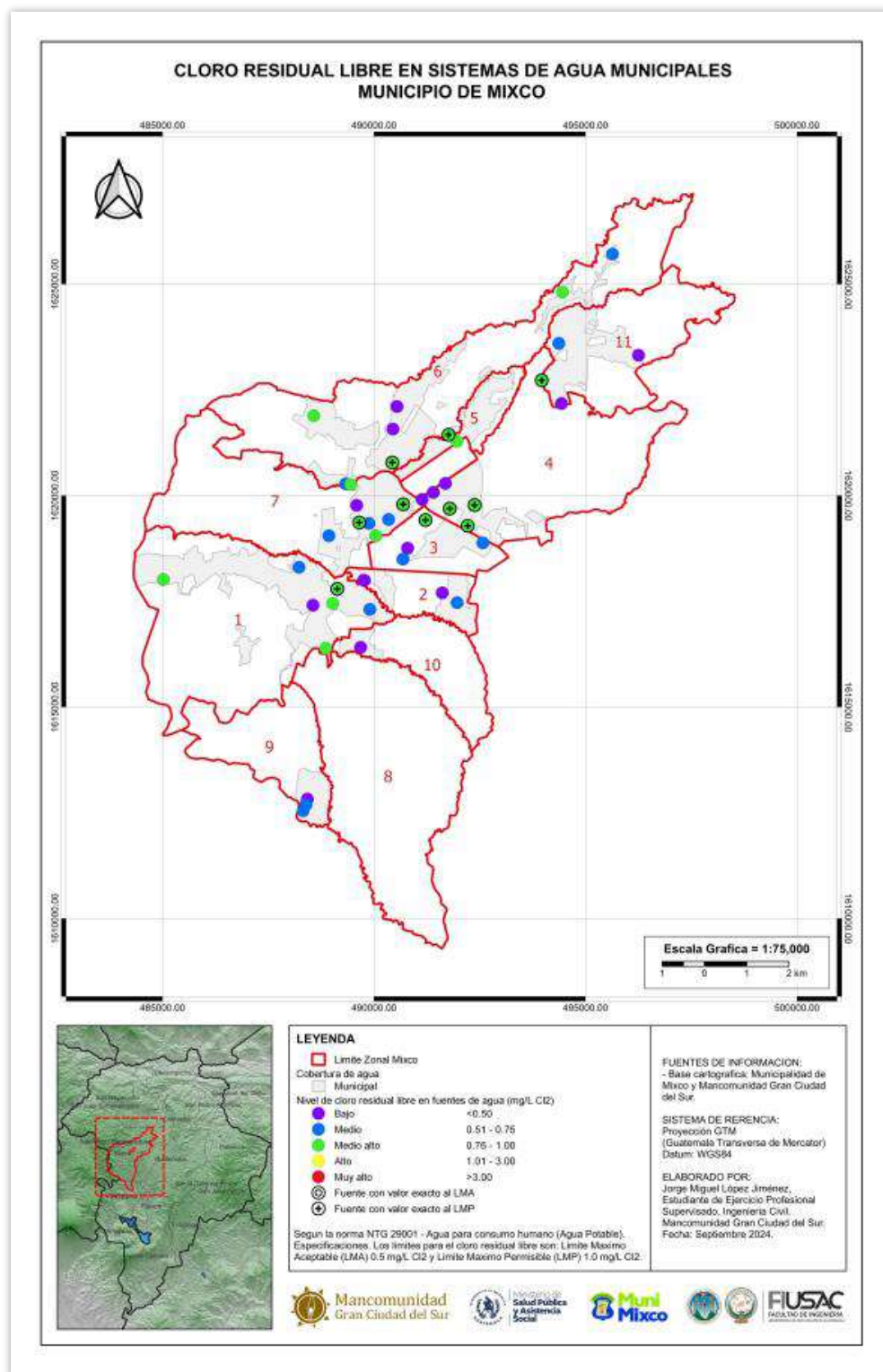
Mapa 28 – Cloro residual libre en sistemas de agua municipales
