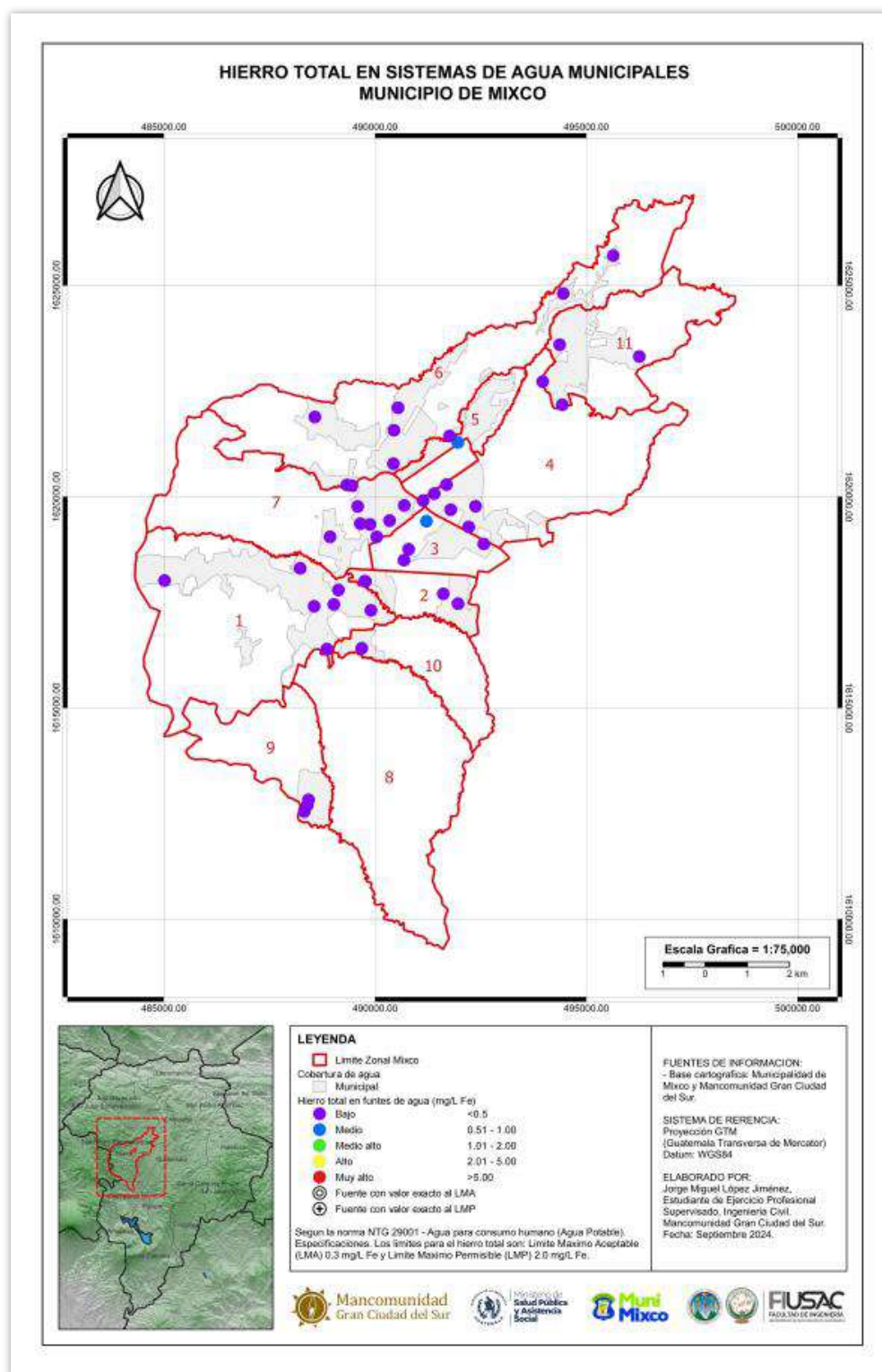
Mapa 30 – Hierro total disuelto en sistemas de agua municipales
