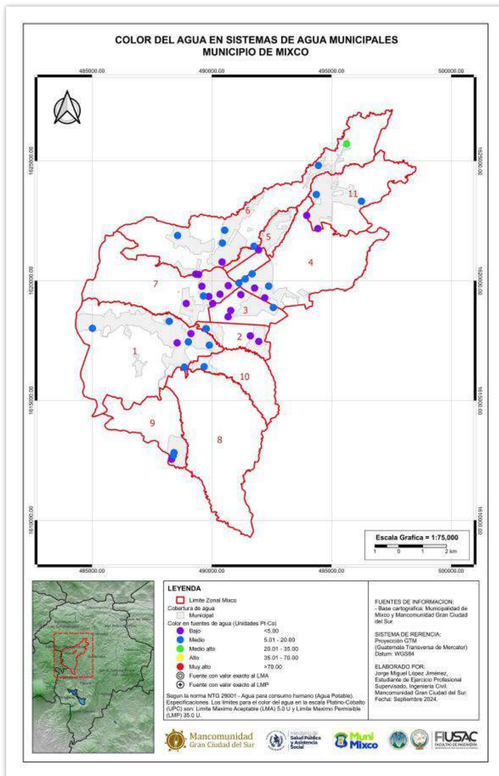
Mapa 29 – Color del agua en sistemas de agua municipales
