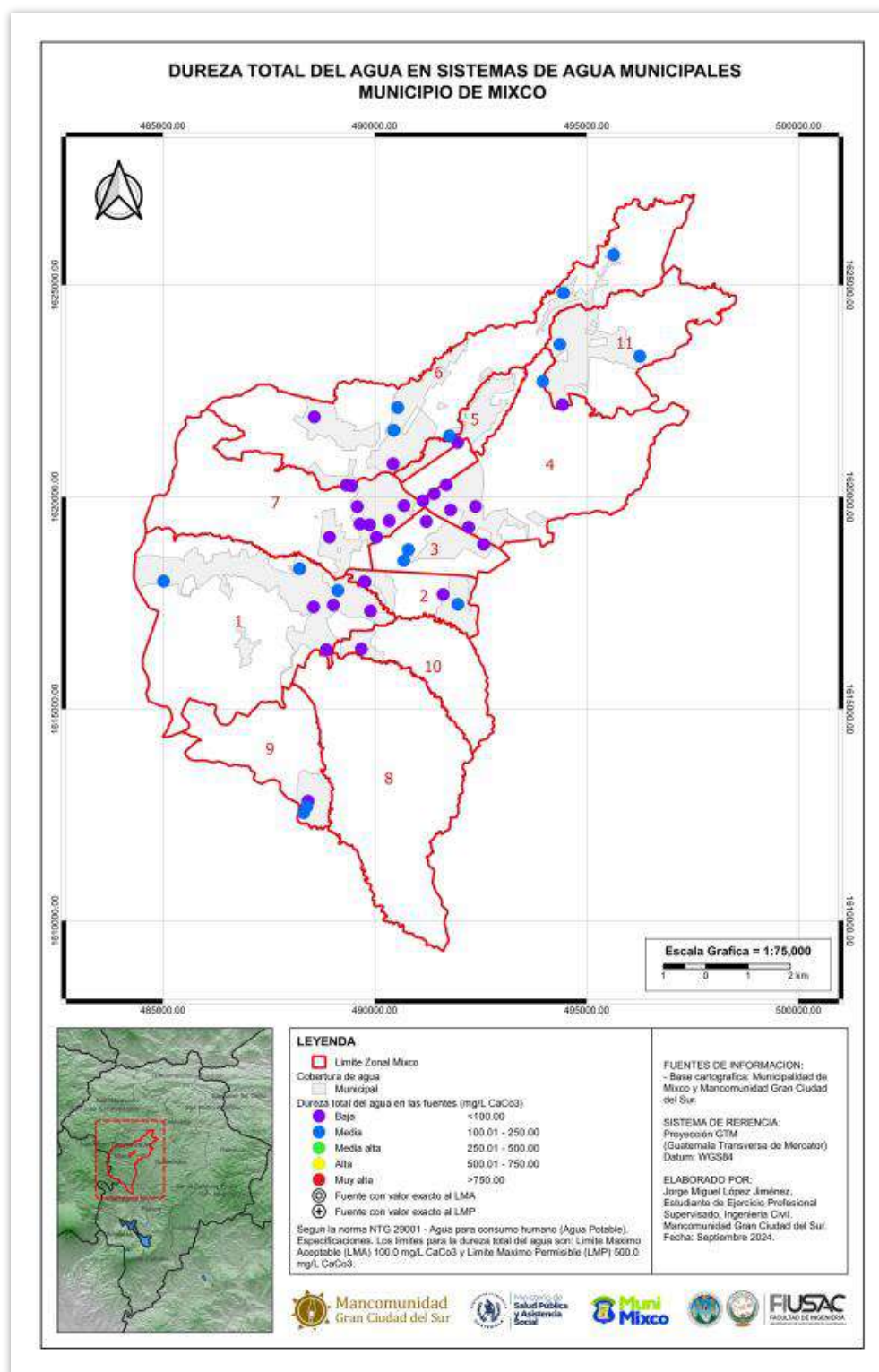
Mapa 37 – Dureza total del agua en sistemas de agua municipales
