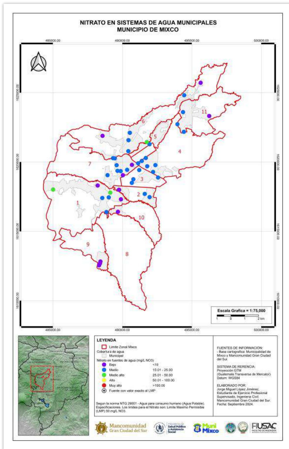
Mapa 32 – Nitrato disuelto en sistemas de agua municipales
